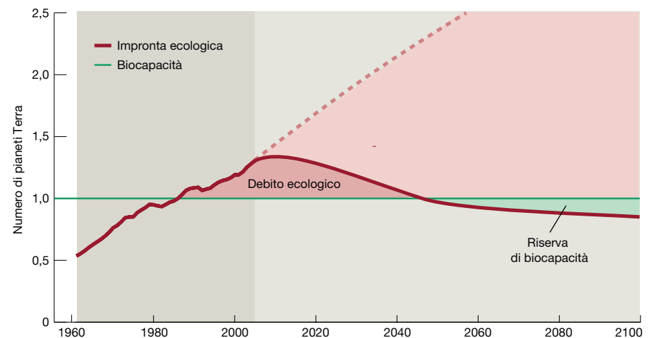
Fig. 32: RITORNO ALLA SOSTENIBILITÀ
