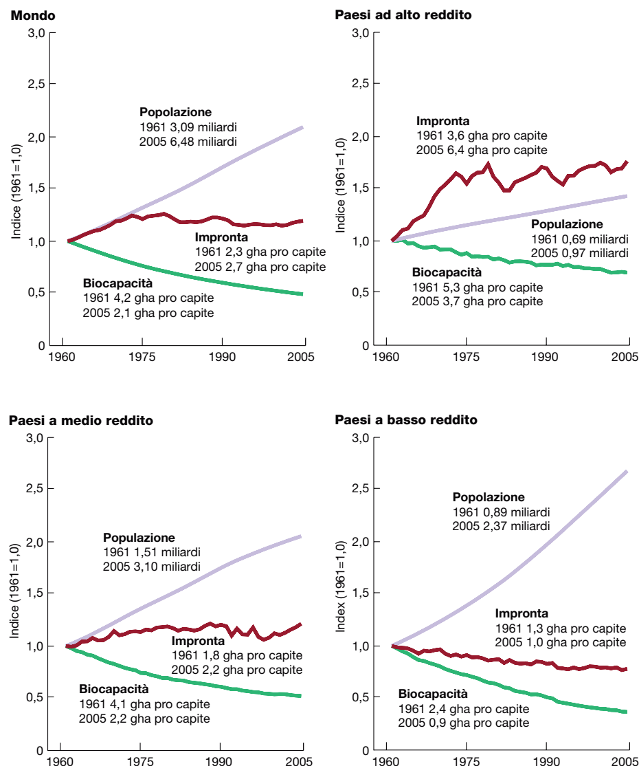
Fig. 40: IMPRONTA ECOLOGICA, BIOCAPACITÀ E POPOLAZIONE RIPORTATE PER IL MONDO E I PAESI AD ALTO, MEDIO E BASSO REDDITO, 1961-2005
