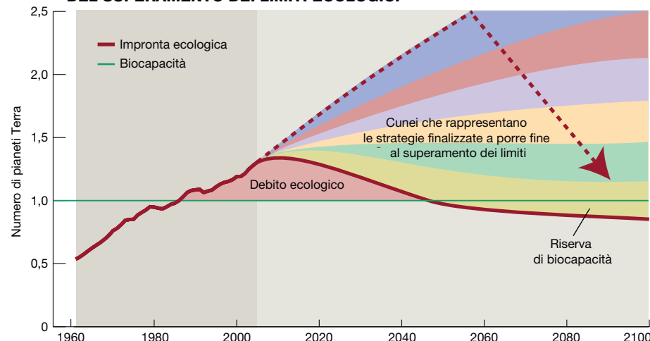
Fig. 34: CUNEI DI SOSTENIBILITÀ E CESSAZIONE DEL SUPERAMENTO DEI LIMITI ECOLOGICI
