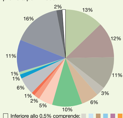
Fig. 37: PRINCIPALI CUNEI ENERGETICI, percentuale di energia fornita o risparmiata nella domanda energetica prevista per il 2050.
