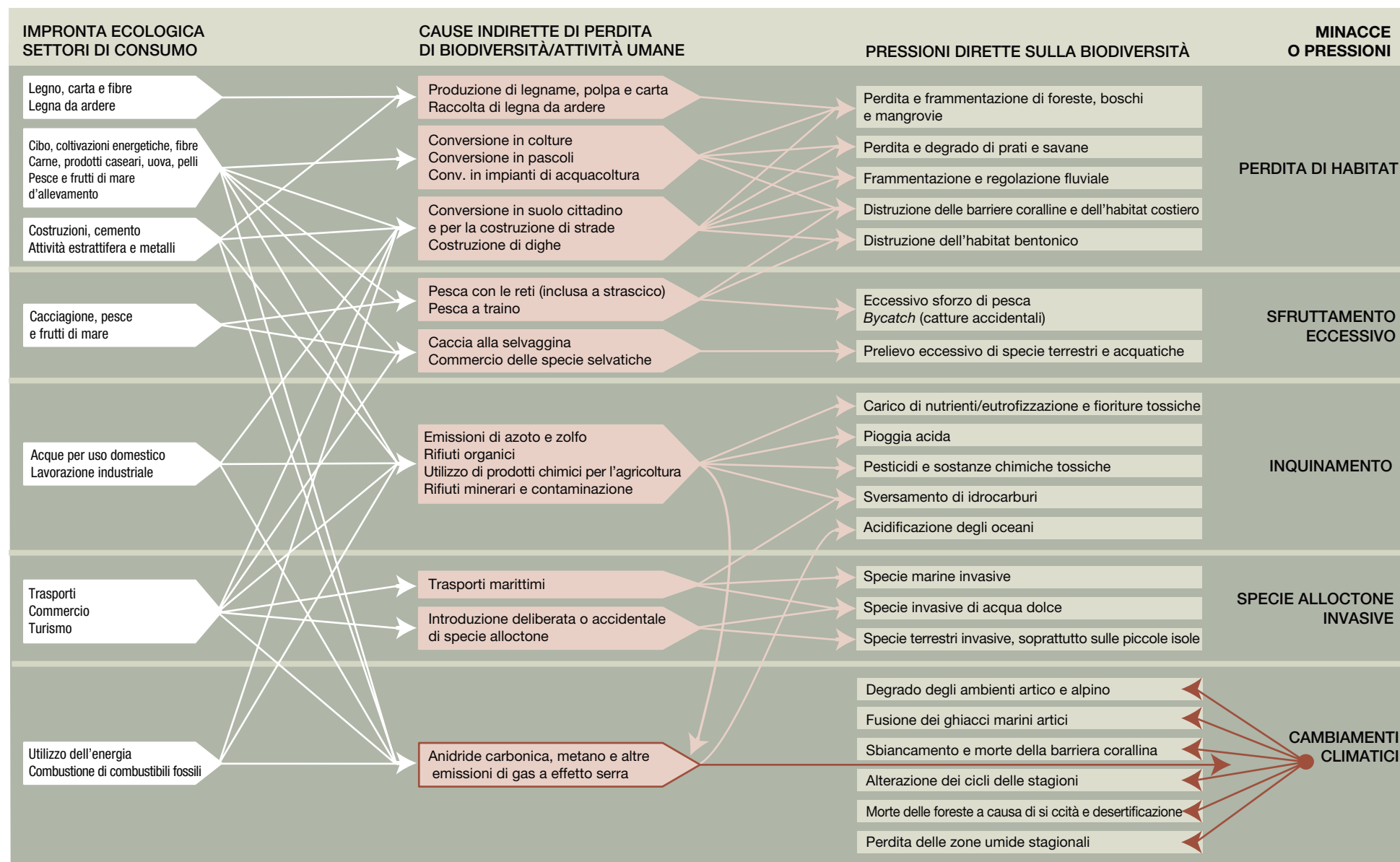
Fig. 4: PERDITA DI BIODIVERSITÀ, PRESSIONE UMANA E IMPRONTA ECOLOGICA , relazioni causa/effetto
