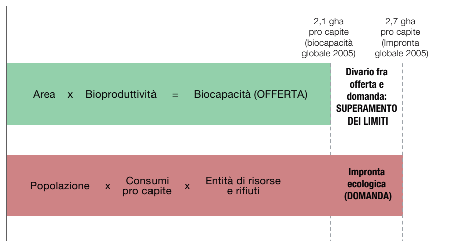
Fig. 33: IMPRONTA E FATTORI DI BIOCAPACITÀ CHE DETERMINANO IL SUPERAMENTO DEI LIMITI ECOLOGICI
